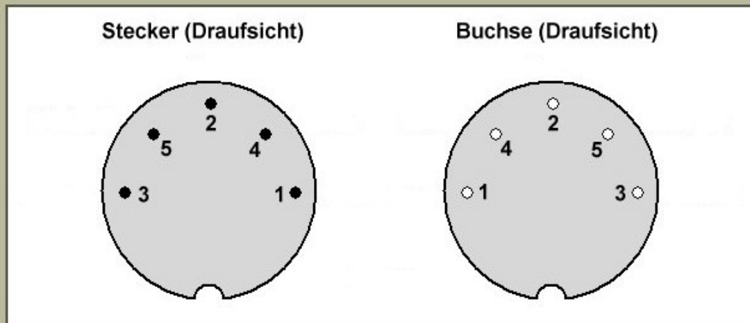
Anschlußbelegung DIN-Stecker und -buchse
